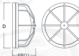
BLH4 D - 15" PROJ. - 7"
