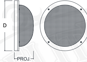
BLH1 D-15" PROJ.-5.75"
