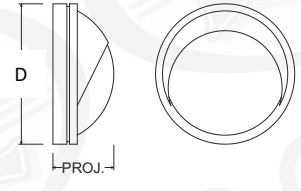
BLHB1 D - 10" PROJ. - 4"
