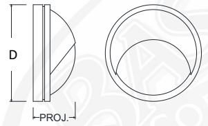
BLHB2 D - 10" PROJ. - 4"
