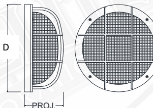
BLH3 D - 15" PROJ. - 6.5"
