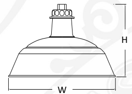
W5134 H-9.5" W-13"
