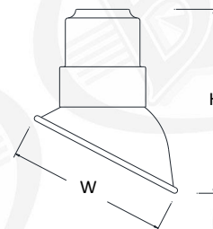
A807 H - 8" W - 7"
