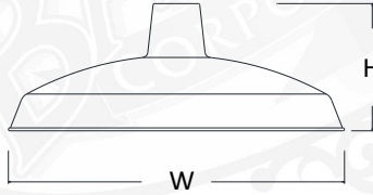
MW529 H-11" W-29"
