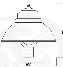
IW20 H-17" W-20" F-3"
