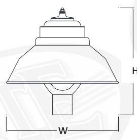
IW20 H-17" W-20" F-3"
