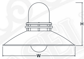
UDP18 H - 8.5" W - 18" UDP218 H - 10.5" W - 18"
