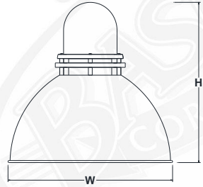
UDP16 H - 13.5" W - 16" UDP216 H - 15.5" W - 16"
