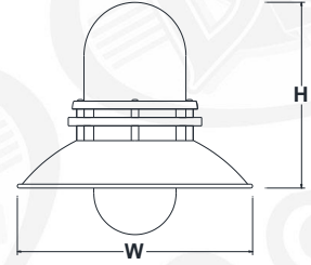
UDP12 H - 7.5" W - 12" UDP212 H - 9.5" W - 12"
