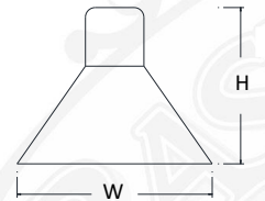
HV108 H-8" W-10"
