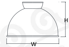
HVF18 H-12" W-18"
