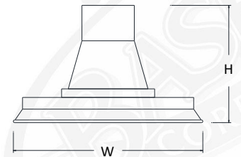
UR14 H-8.75" W-14"
