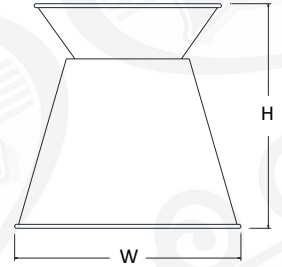
UDC14 H - 14.25" W - 14.5"
