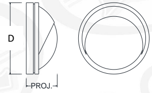
BLHB1 D - 10" PROJ. – 4.5"
