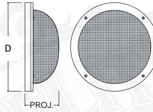
BLH1 D-15" PROJ.-5.75"
