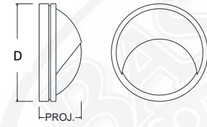
BLHB2 D - 10" PROJ. - 4.5"
