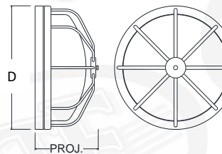
BLH4 D-15" PROJ.-7.5"
