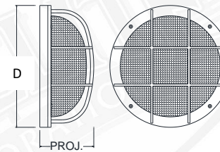
BLH3 D-15" PROJ.-6.5"
