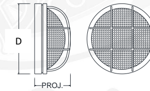
BLHB4 D - 10" PROJ. – 5.25"
