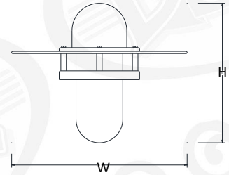
FL3 H-9.5" W-12"
