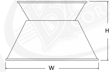
UDC16 H - 10" W - 16"
