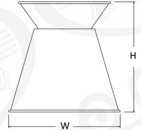
UDC14 H - 14.25" W - 14.5"
